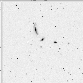
Arp_290_15x15
