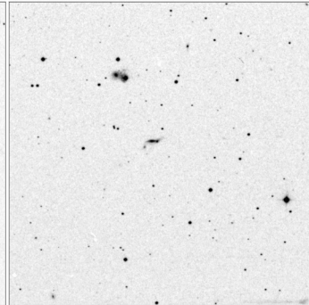
Arp_63_15x15
