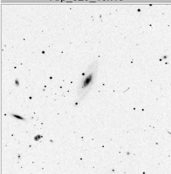
Arp_333_15x15
