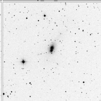
Arp_166_15x15
