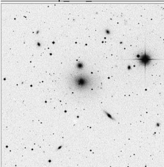
Arp_229_15x15
