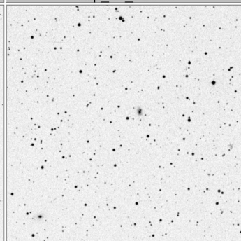
Arp_52_15x15
