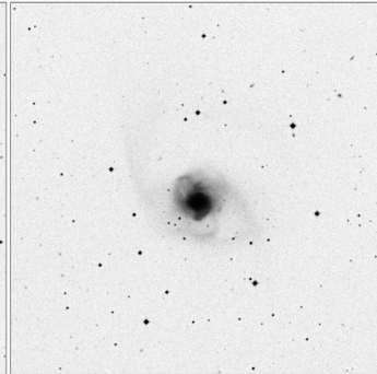
Arp_222_15x15
