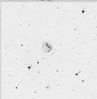
Arp_5_15x15
