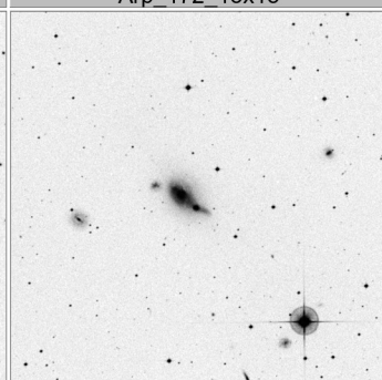
Arp_176_15x15
