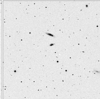
Arp_303_15x15
