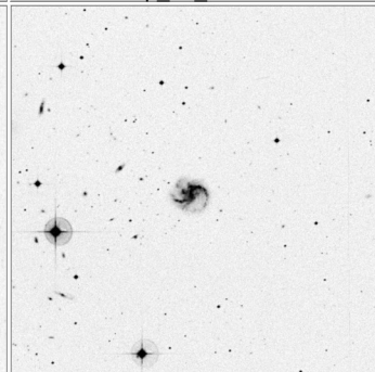
Arp_19_15x15
