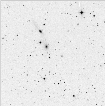
Arp_101_15x15
