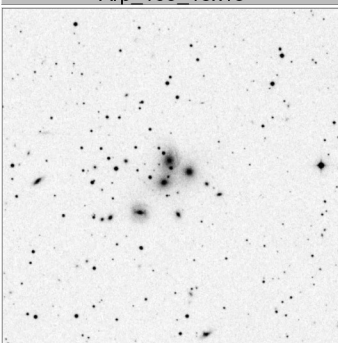
Arp_113_15x15
