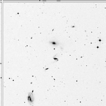
Arp_332_15x15
