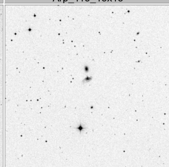
Arp_119_15x15
