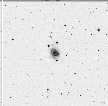
Arp_28_15x15
