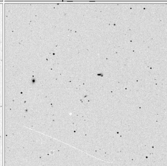
Arp_148_15x15
