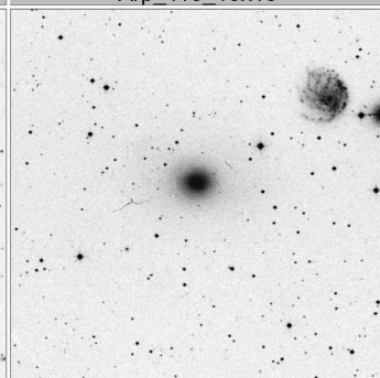
Arp_114_15x15
