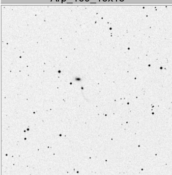
Arp_173_15x15
