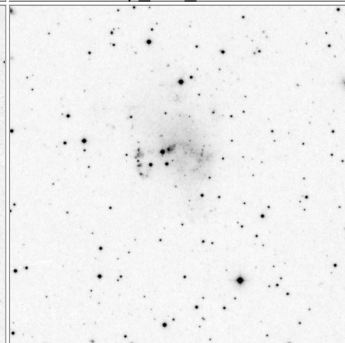
Arp_268_15x15
