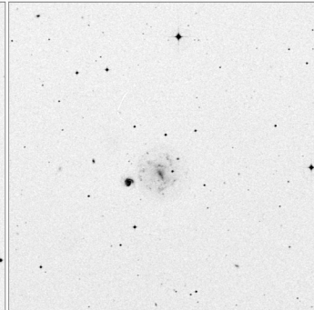
Arp_4_15x15
