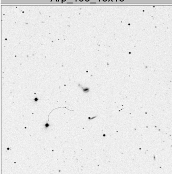
Arp_197_15x15
