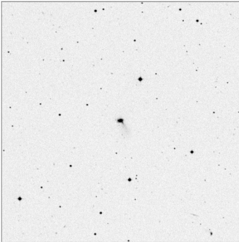
Arp_161_15x15
