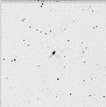
Arp_193_15x15
