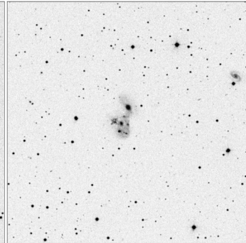
Arp_143_15x15
