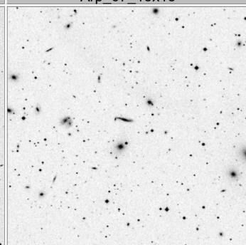
Arp_71_15x15
