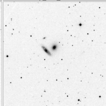
Arp_307_15x15
