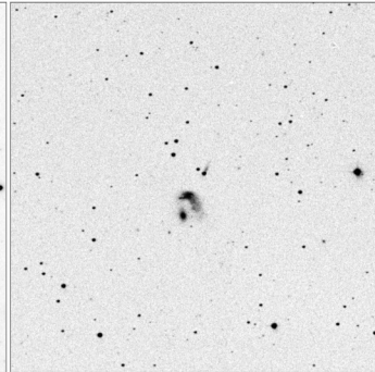
Arp_142_15x15
