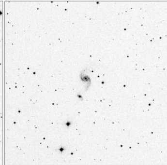
Arp_82_15x15
