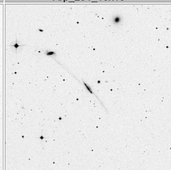
Arp_295_15x15
