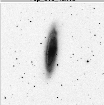
Arp_317_15x15
