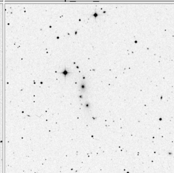
Arp_330_15x15
