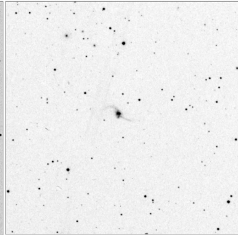
Arp_243_15x15
