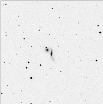
Arp_121_15x15
