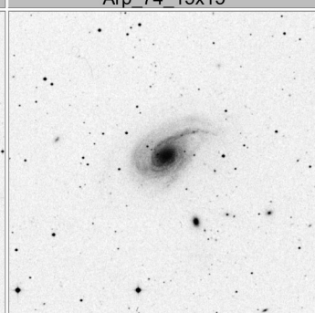
Arp_78_15x15
