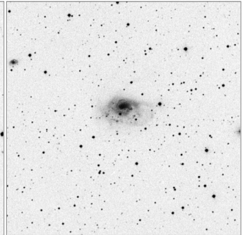
Arp_184_15x15
