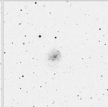
Arp_3_15x15
