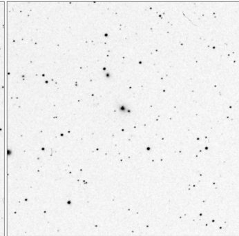
Arp_103_15x15
