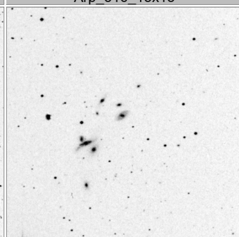
Arp_320_15x15
