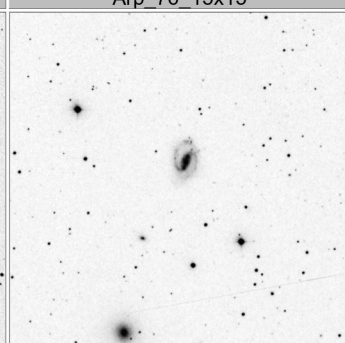
Arp_80_15x15
