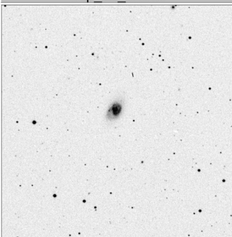
Arp_49_15x15
