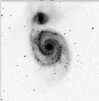
Arp_85_15x15
