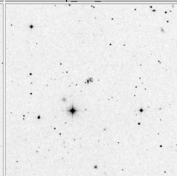
Arp_147_15x15
