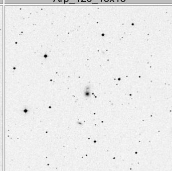
Arp_130_15x15
