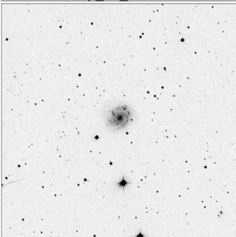
Arp_38_15x15
