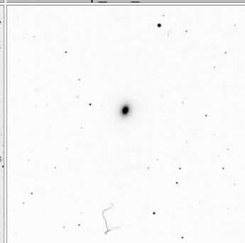
Arp_168_15x15
