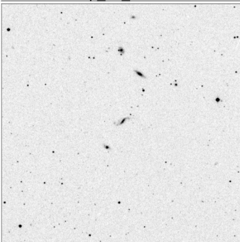
Arp_33_15x15
