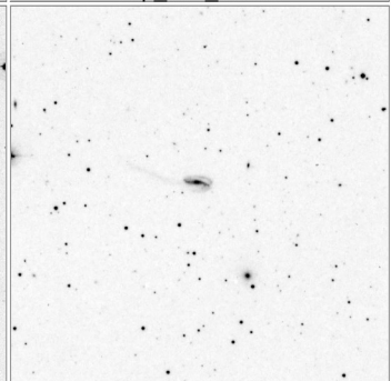
Arp_188_15x15
