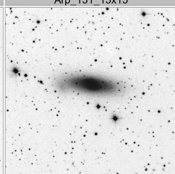
Arp_135_15x15
