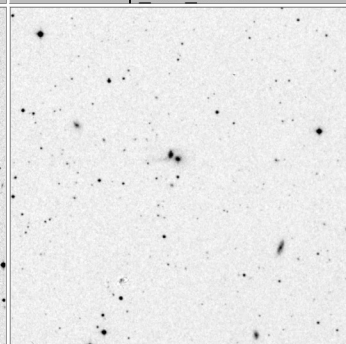
Arp_191_15x15
