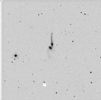
Arp_242_15x15
