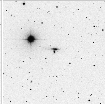
Arp_282_15x15
