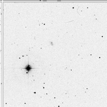
Arp_211_15x15
