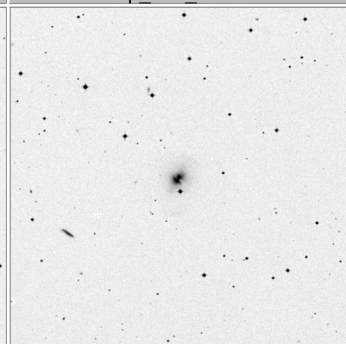
Arp_231_15x15
