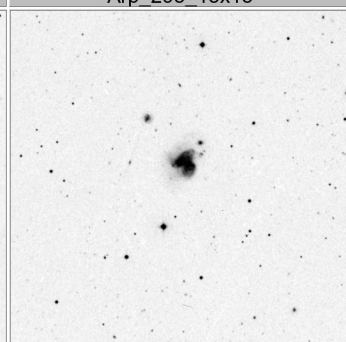
Arp_299_15x15
