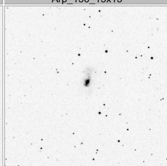
Arp_160_15x15
