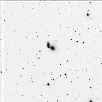
Arp_91_15x15
