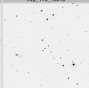
Arp_179_15x15
