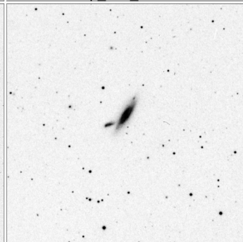
Arp_280_15x15
