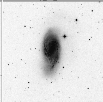
Arp_16_15x15
