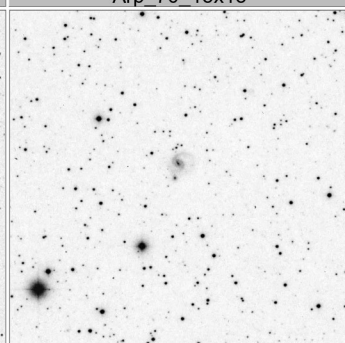
Arp_74_15x15
