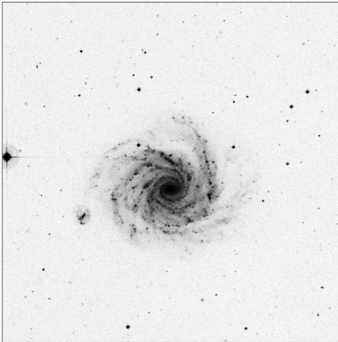
Arp_41_15x15
