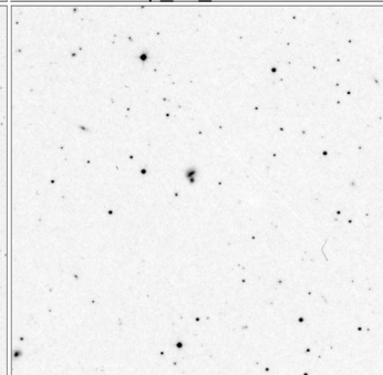
Arp_40_15x15
