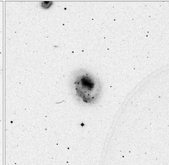
Arp_23_15x15
