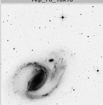
Arp_77_15x15
