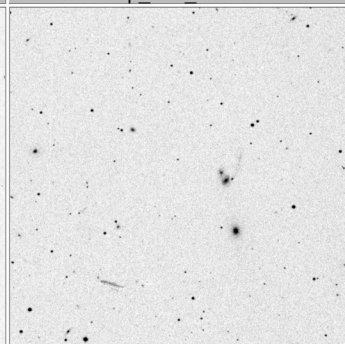
Arp_190_15x15
