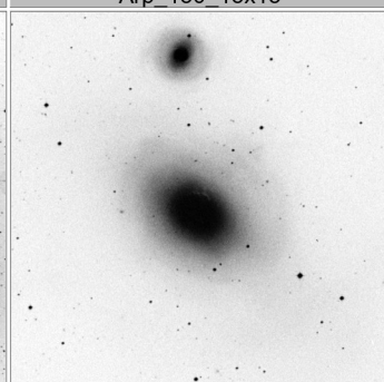
Arp_154_15x15
