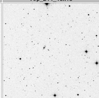
Arp_218_15x15
