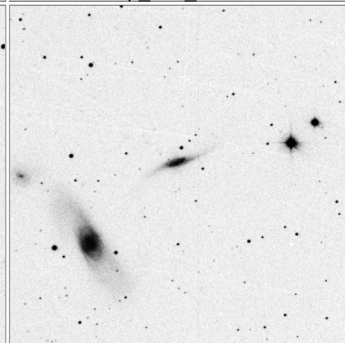
Arp_286_15x15
