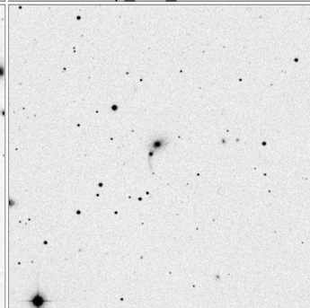
Arp_106_15x15
