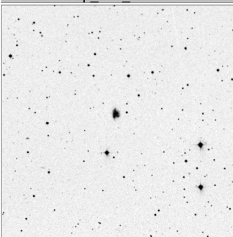
Arp_209_15x15
