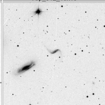
Arp_316_15x15
