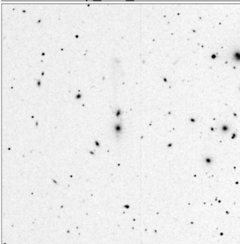
Arp_105_15x15
