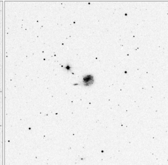
Arp_24_15x15
