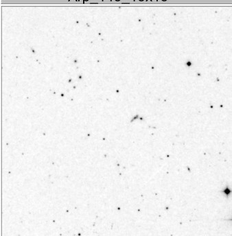
Arp_149_15x15
