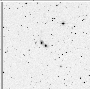
Arp_112_15x15
