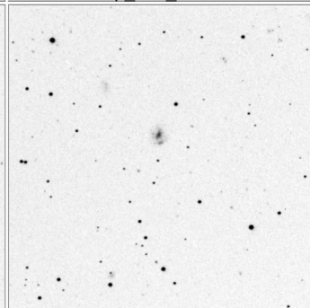
Arp_306_15x15
