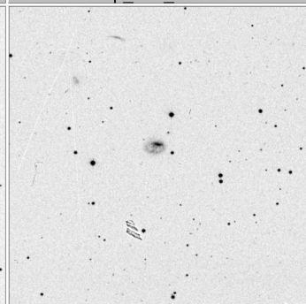
Arp_291_15x15
