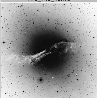
Arp_153_15x15
