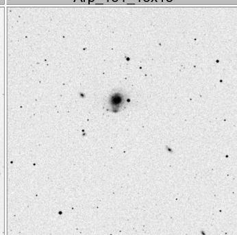
Arp_155_15x15
