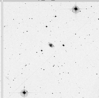
Arp_20_15x15
