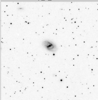
Arp_9_15x15
