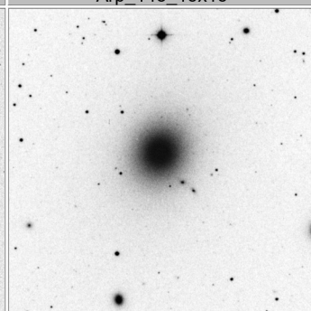
Arp_152_15x15
