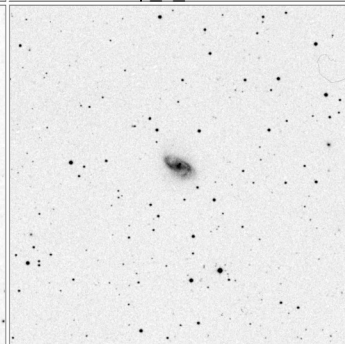
Arp_12_15x15
