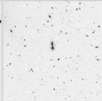
Arp_302_15x15
