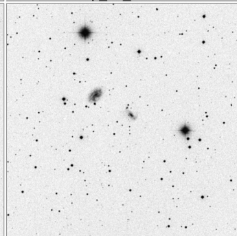
Arp_46_15x15
