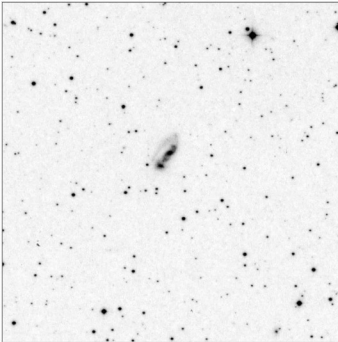
Arp_81_15x15
