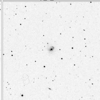
Arp_10_15x15
