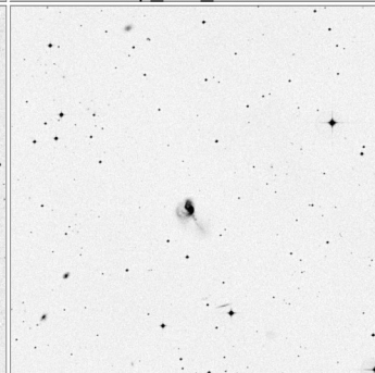
Arp_186_15x15
