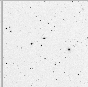
Arp_64_15x15
