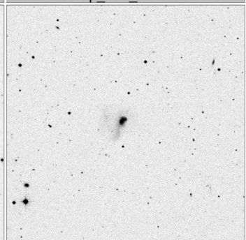
Arp_192_15x15
