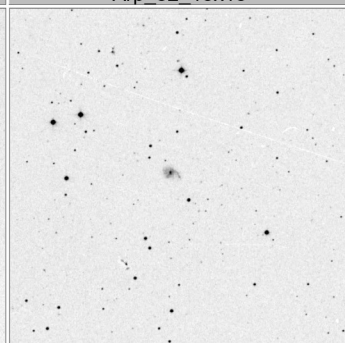
Arp_56_15x15
