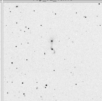
Arp_97_15x15
