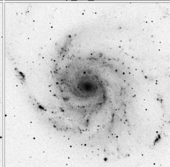
Arp_26_15x15
