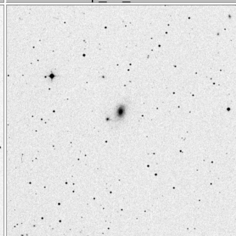
Arp_92_15x15
