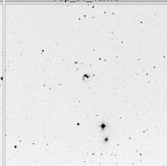
Arp_55_15x15
