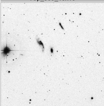
Arp_313_15x15
