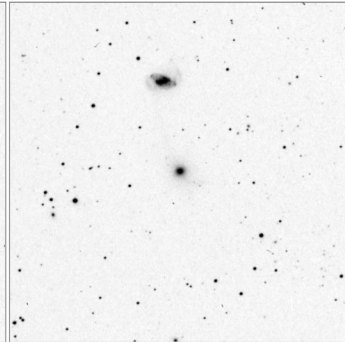
Arp_104_15x15
