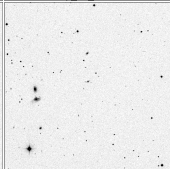
Arp_88_15x15
