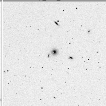
Arp_228_15x15
