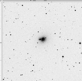
Arp_167_15x15
