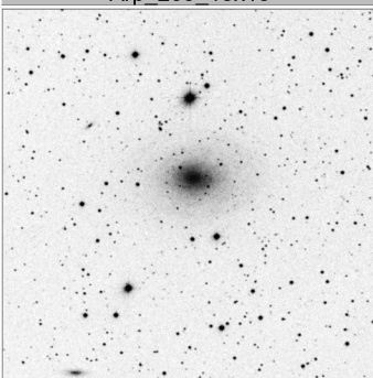
Arp_213_15x15
