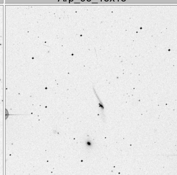
Arp_100_15x15
