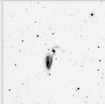
Arp_84_15x15
