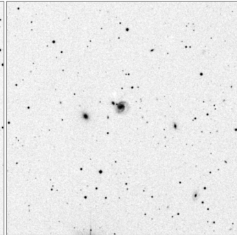
Arp_182_15x15
