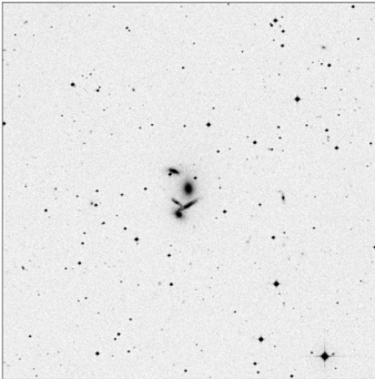
Arp_321_15x15
