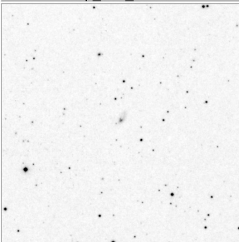
Arp_265_15x15
