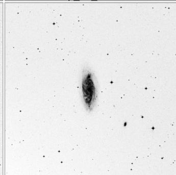
Arp_14_15x15
