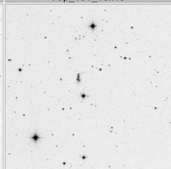
Arp_195_15x15
