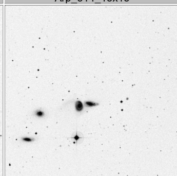
Arp_318_15x15
