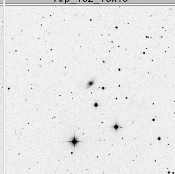
Arp_156_15x15
