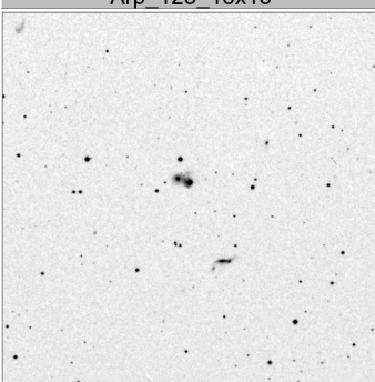
Arp_129_15x15
