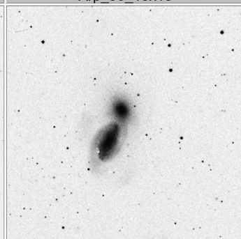
Arp_94_15x15
