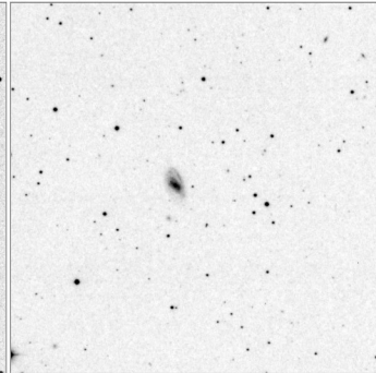
Arp_44_15x15
