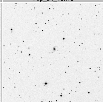
Arp_58_15x15
