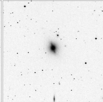
Arp_162_15x15
