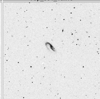
Arp_335_15x15
