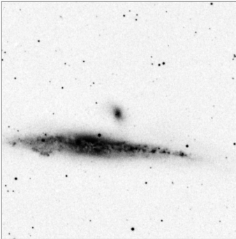
Arp_281_15x15
