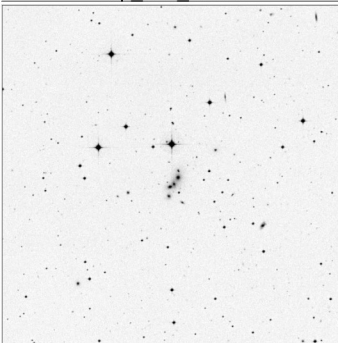
Arp_325_15x15
