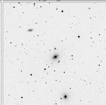
Arp_292_15x15
