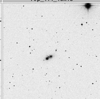
Arp_118_15x15
