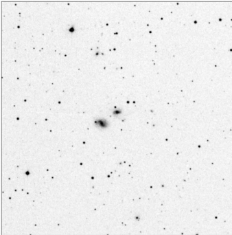
Arp_181_15x15
