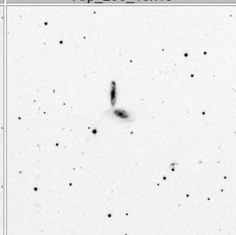
Arp_294_15x15
