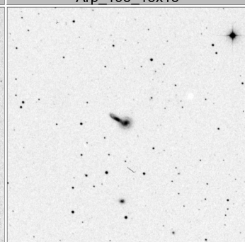
Arp_199_15x15
