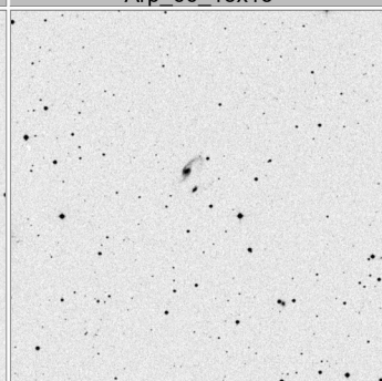
Arp_70_15x15
