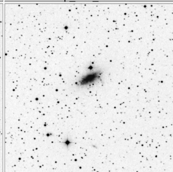
Arp_210_15x15
