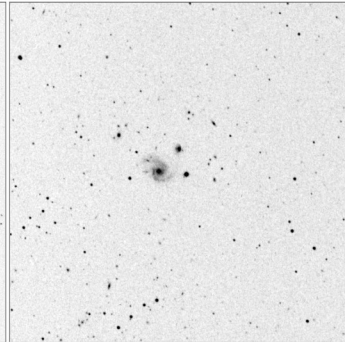
Arp_42_15x15
