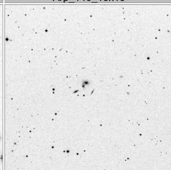
Arp_150_15x15
