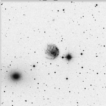
Arp_25_15x15
