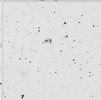
Arp_274_15x15
