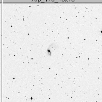
Arp_180_15x15
