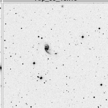
Arp_72_15x15
