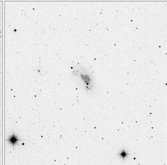
Arp_264_15x15
