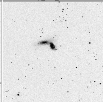
Arp_270_15x15
