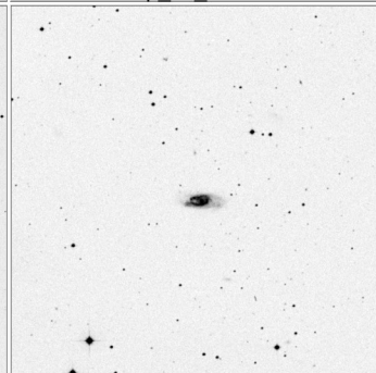
Arp_15_15x15
