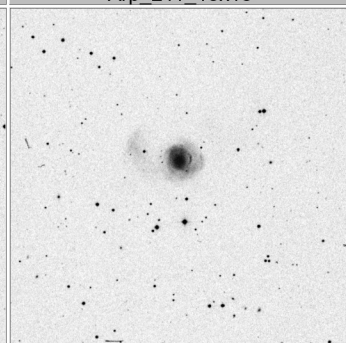
Arp_215_15x15
