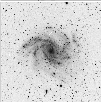
Arp_29_15x15
