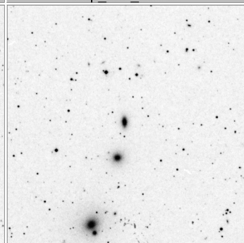
Arp_331_15x15
