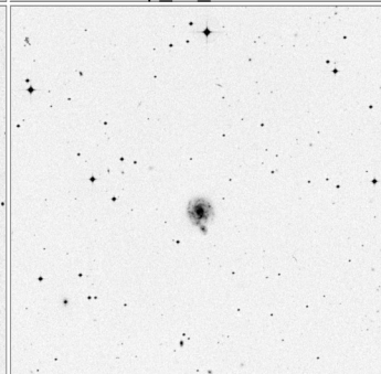
Arp_39_15x15
