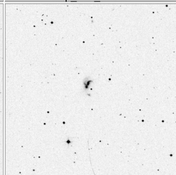
Arp_111_15x15
