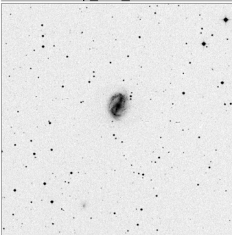
Arp_185_15x15
