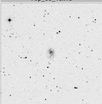
Arp_69_15x15
