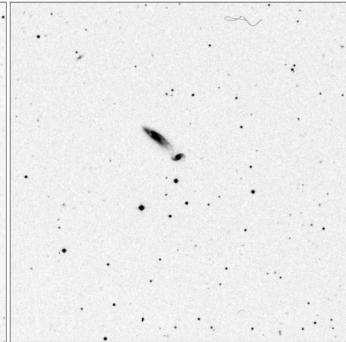
Arp_83_15x15
