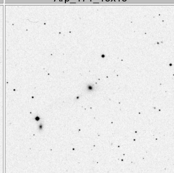
Arp_175_15x15
