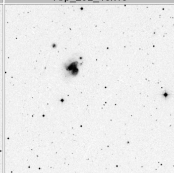
Arp_296_15x15
