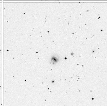
Arp_67_15x15
