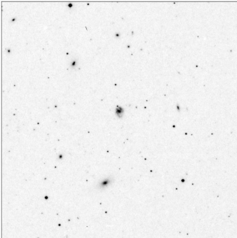
Arp_21_15x15
