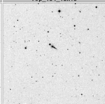
Arp_198_15x15
