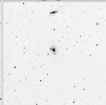
Arp_288_15x15
