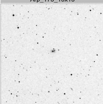
Arp_177_15x15
