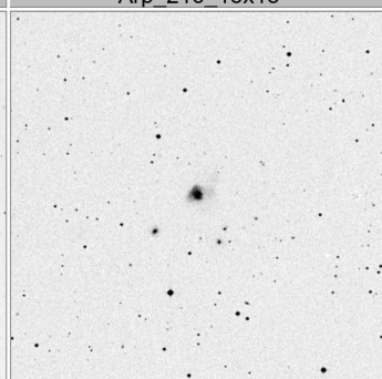
Arp_220_15x15
