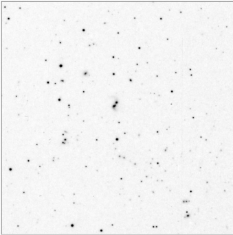
Arp_241_15x15
