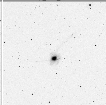
Arp_226_15x15
