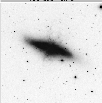
Arp_337_15x15
