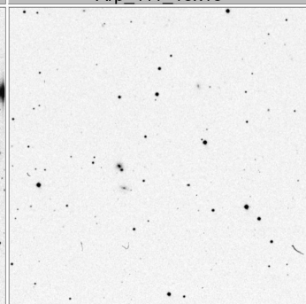
Arp_115_15x15
