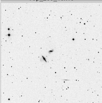
Arp_293_15x15
