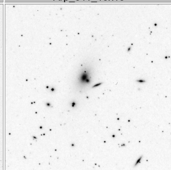
Arp_315_15x15
