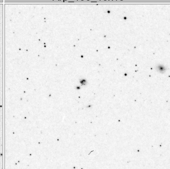
Arp_194_15x15
