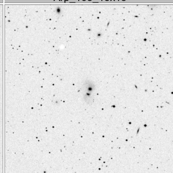
Arp_172_15x15
