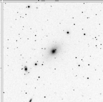
Arp_232_15x15
