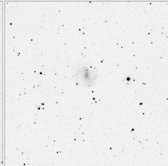
Arp_2_15x15
