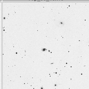
Arp_54_15x15
