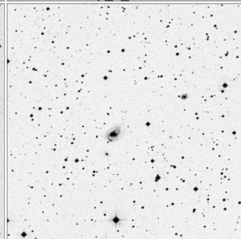
Arp_7_15x15
