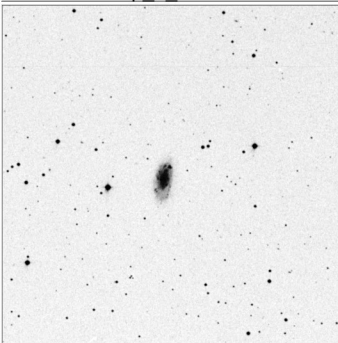
Arp_13_15x15
