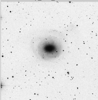
Arp_225_15x15
