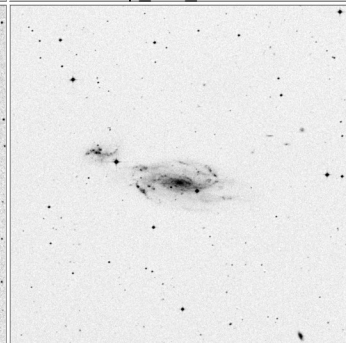
Arp_279_15x15
