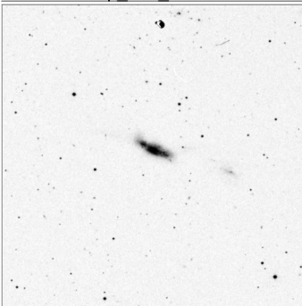
Arp_205_15x15
