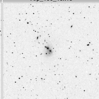
Arp_170_15x15
