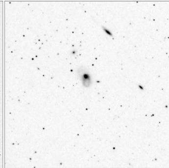
Arp_224_15x15
