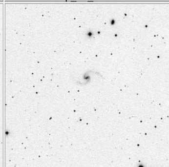
Arp_31_15x15
