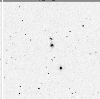
Arp_87_15x15
