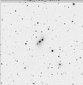
Arp_169_15x15
