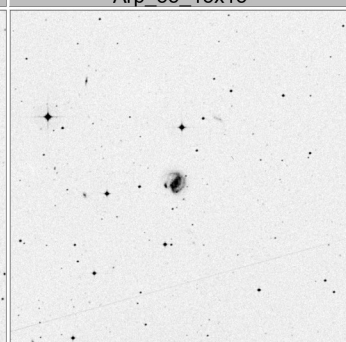
Arp_59_15x15
