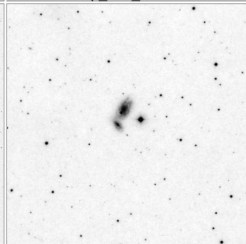
Arp_276_15x15
