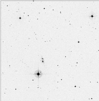
Arp_201_15x15
