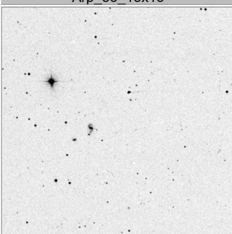
Arp_57_15x15
