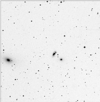
Arp_61_15x15
