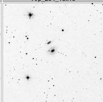
Arp_298_15x15
