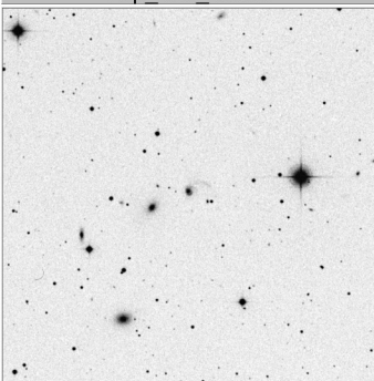
Arp_109_15x15
