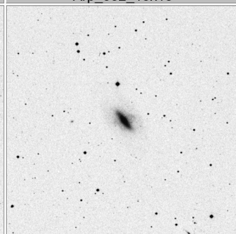
Arp_336_15x15
