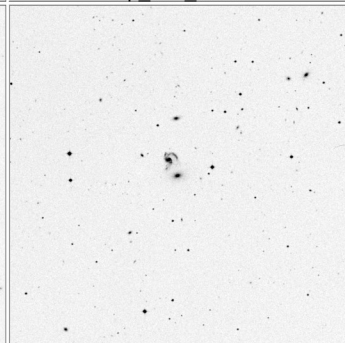
Arp_108_15x15
