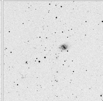
Arp_43_15x15
