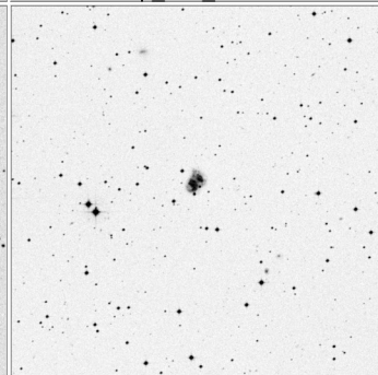
Arp_275_15x15
