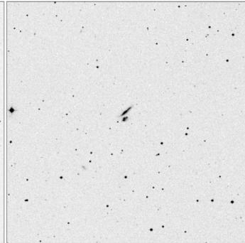
Arp_202_15x15
