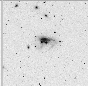
Arp_263_15x15
