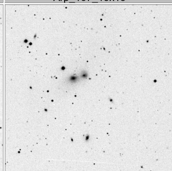
Arp_171_15x15
