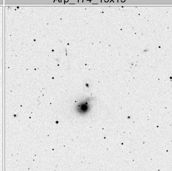
Arp_178_15x15
