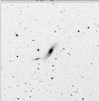
Arp_89_15x15
