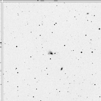
Arp_110_15x15
