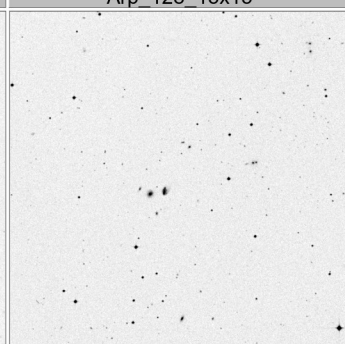
Arp_132_15x15
