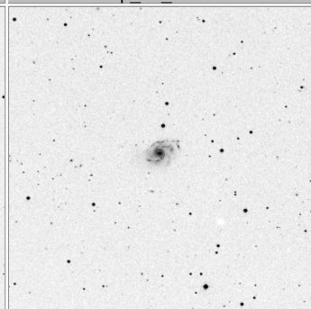
Arp_68_15x15
