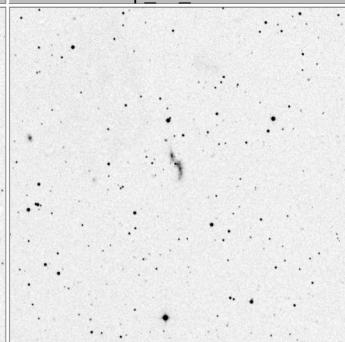
Arp_32_15x15
