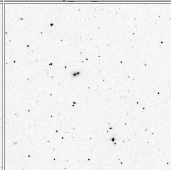
Arp_128_15x15
