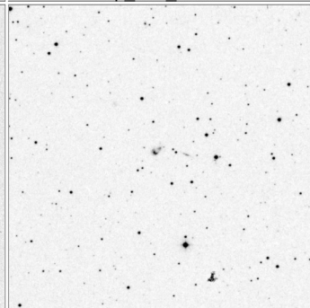
Arp_208_15x15
