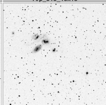
Arp_319_15x15
