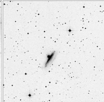
Arp_123_15x15
