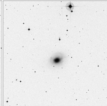
Arp_223_15x15
