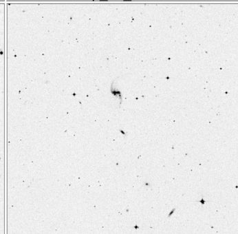
Arp_35_15x15
