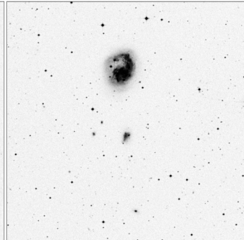
Arp_22_15x15
