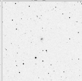
Arp_36_15x15
