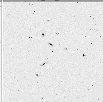
Arp_326_15x15
