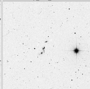
Arp_328_15x15
