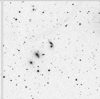
Arp_122_15x15
