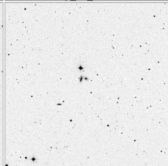
Arp_47_15x15
