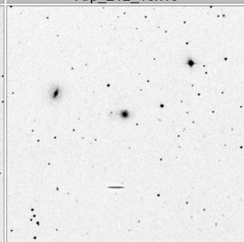
Arp_216_15x15
