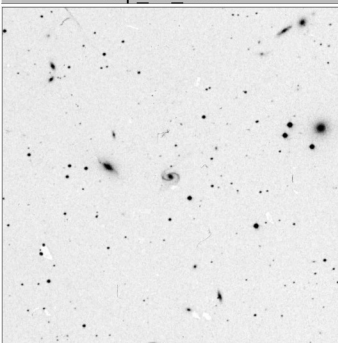
Arp_65_15x15
