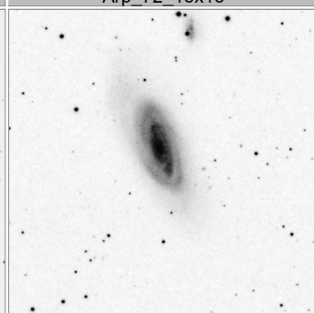
Arp_76_15x15
