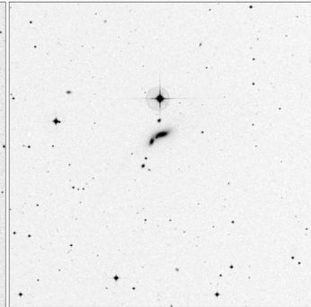
Arp_323_15x15
