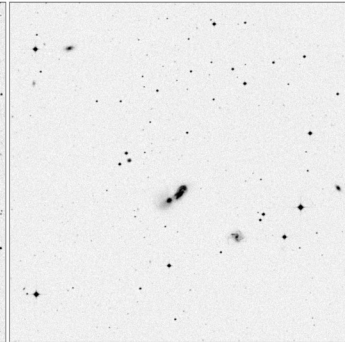
Arp_144_15x15
