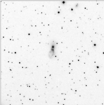
Arp_141_15x15
