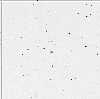
Arp_146_15x15
