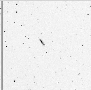
Arp_62_15x15
