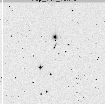
Arp_151_15x15
