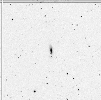
Arp_334_15x15
