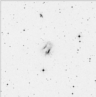
Arp_261_15x15
