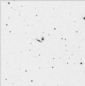
Arp_301_15x15
