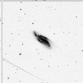
Arp_18_15x15
