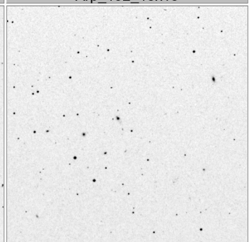
Arp_196_15x15
