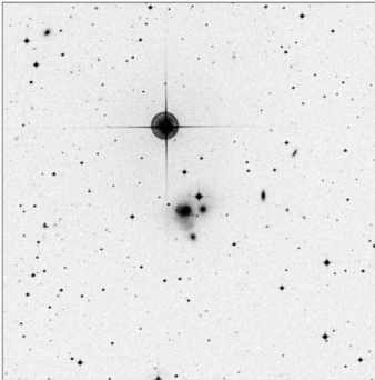
Arp_221_15x15
