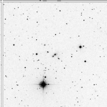
Arp_312_15x15
