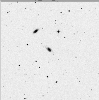
Arp_285_15x15
