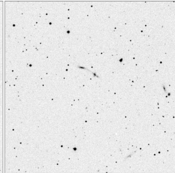
Arp_204_15x15
