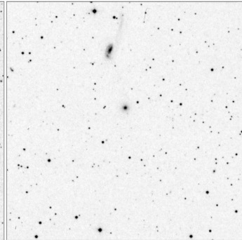
Arp_102_15x15
