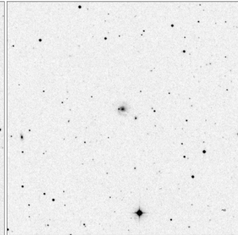
Arp_183_15x15
