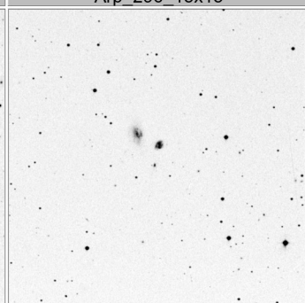
Arp_300_15x15
