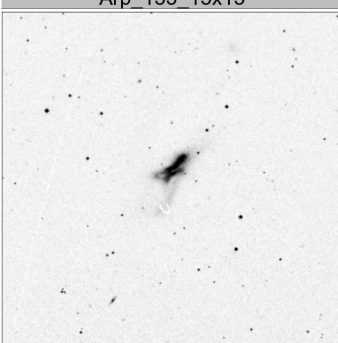
Arp_157_15x15
