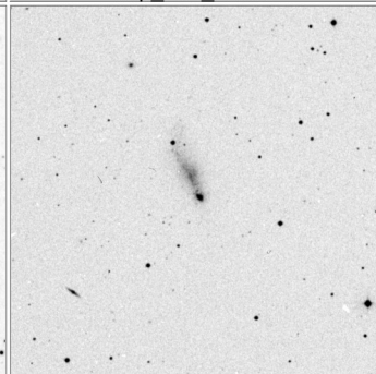
Arp_266_15x15
