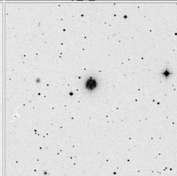
Arp_6_15x15
