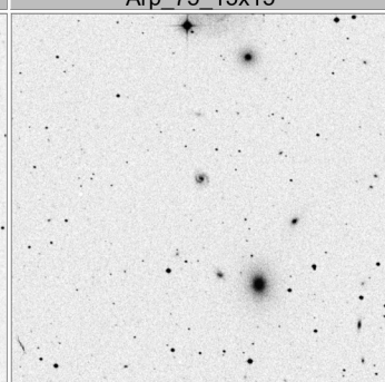
Arp_79_15x15
