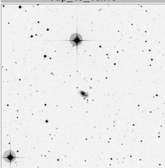
Arp_53_15x15
