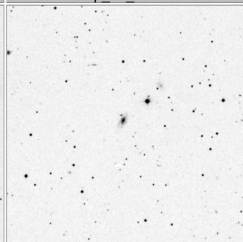
Arp_66_15x15
