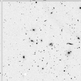
Arp_272_15x15
