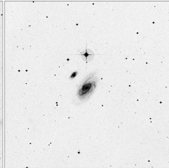
Arp_304_15x15
