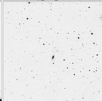
Arp_187_15x15
