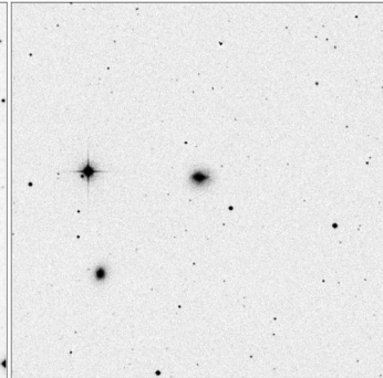
Arp_163_15x15
