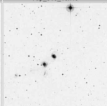
Arp_314_15x15
