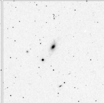
Arp_164_15x15
