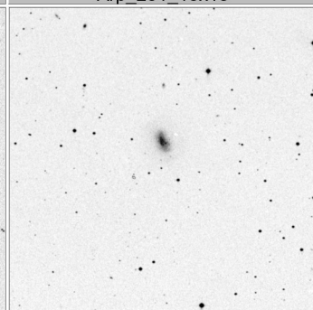
Arp_235_15x15
