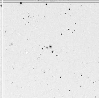
Arp_95_15x15
