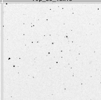
Arp_60_15x15
