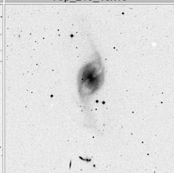
Arp_214_15x15
