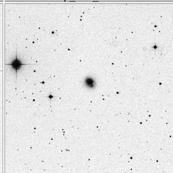
Arp_212_15x15
