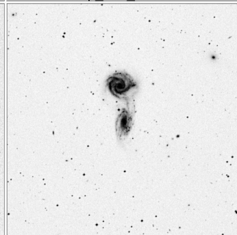
Arp_271_15x15
