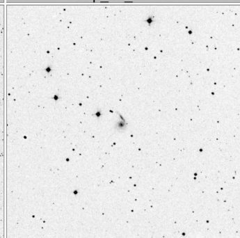
Arp_30_15x15
