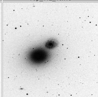
Arp_116_15x15
