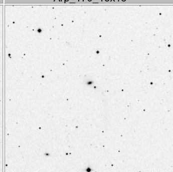
Arp_174_15x15
