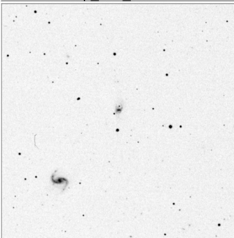
Arp_305_15x15
