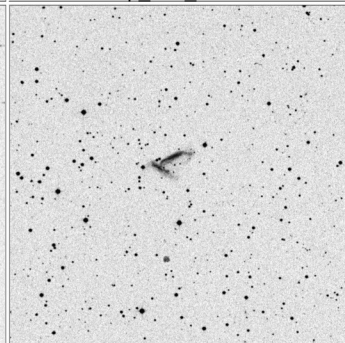
Arp_278_15x15
