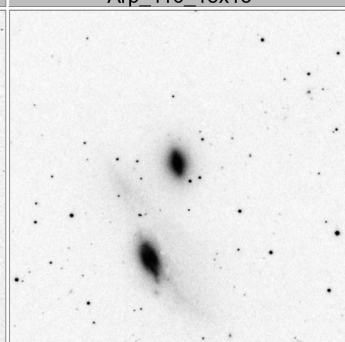
Arp_120_15x15
