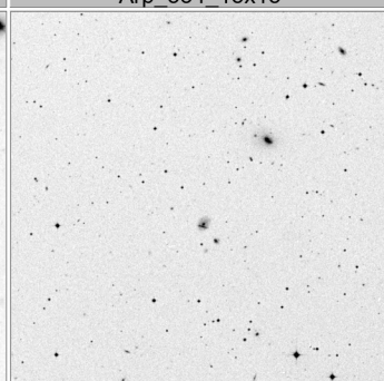
Arp_338_15x15
