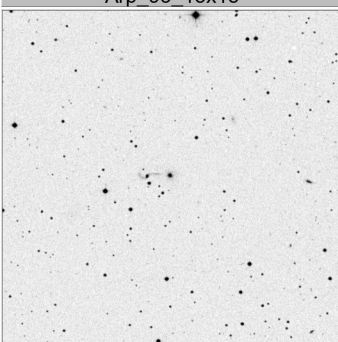
Arp_98_15x15
