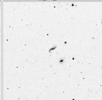
Arp_34_15x15
