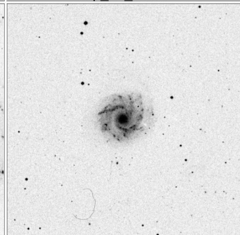
Arp_27_15x15
