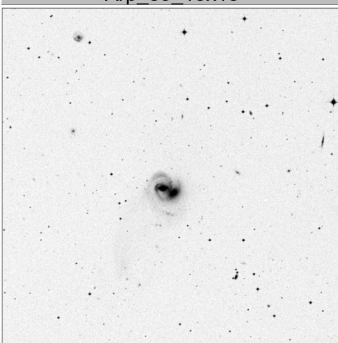
Arp_93_15x15
