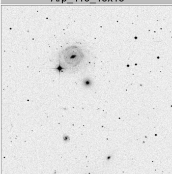
Arp_117_15x15
