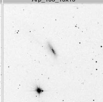
Arp_159_15x15
