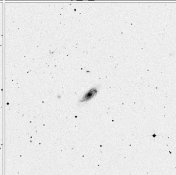
Arp_8_15x15
