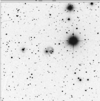
Arp_145_15x15
