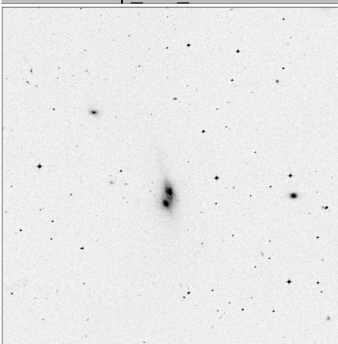
Arp_309_15x15
