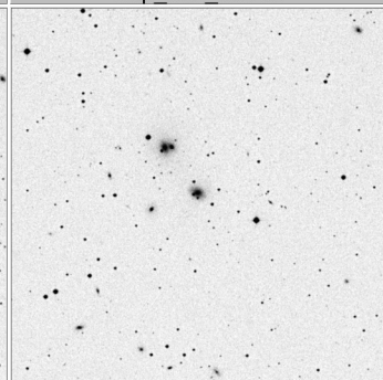
Arp_311_15x15
