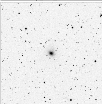
Arp_165_15x15
